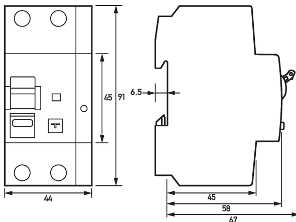
Dibujos acotados DRCBO 4 tipo B+, 1 polo + N (Vista de grupos)
