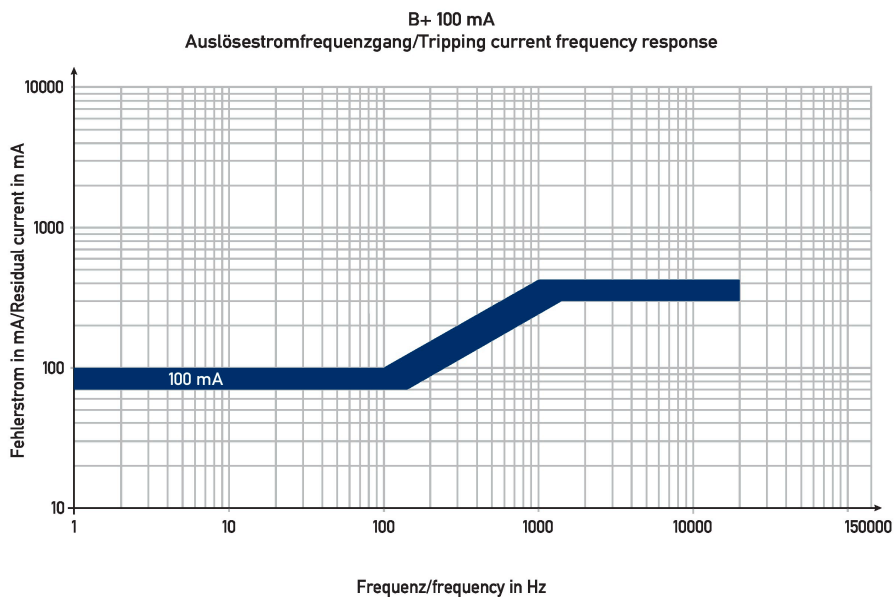
Curva característica B+ 100 mA
