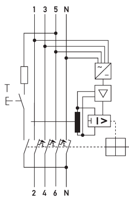
Esquema de conexiones DRCBO 4 tipo B+, 1 polo + N
