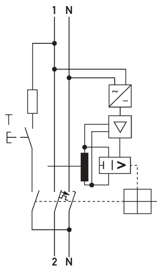
Anschlussschema DRCBO 4 Typ B SK, 1+N-polig
