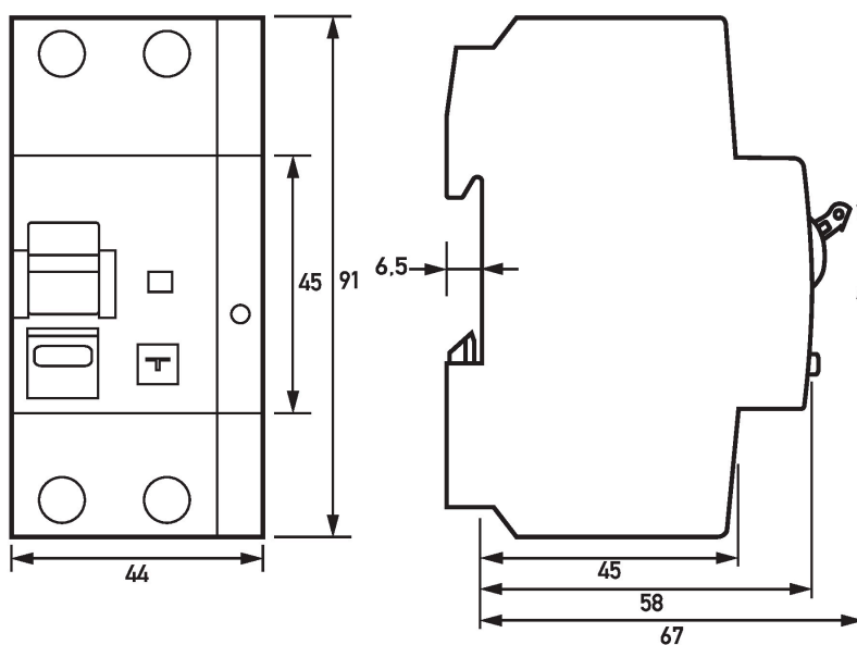
Maßzeichnung DRCBO 4 Typ B SK, einpolig+N (Gruppenansicht)
