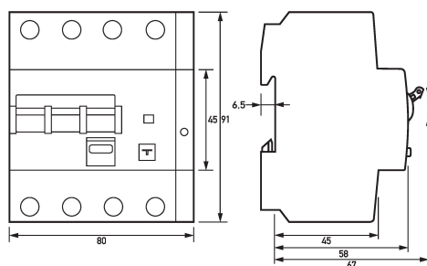
Maßzeichnung FI-/LS-Kombinationen DRCBO 4 HP, 3+N-polig
