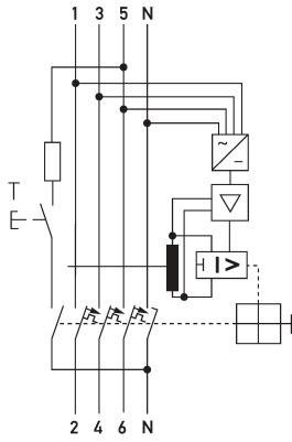
Schaltungsbeispiel FI-/LS-Kombinationen DRCBO 4 HP, 3+N-polig
