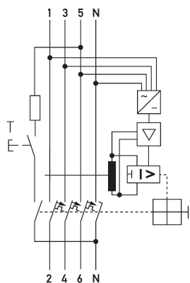
Schaltungsbeispiel FI-/LS-Kombinationen DRCBO 4 PV, 3+N-polig
