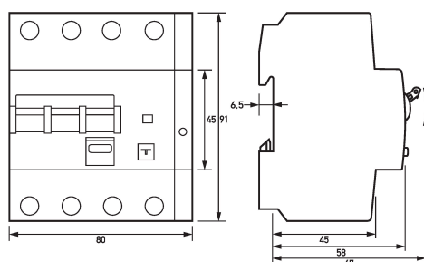
Maßzeichnung FI-/LS-Kombinationen DRCBO 4 PV, 3+N-polig
