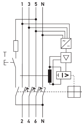
Anschlussschema DRCBO 4 PV, 3+N-polig
