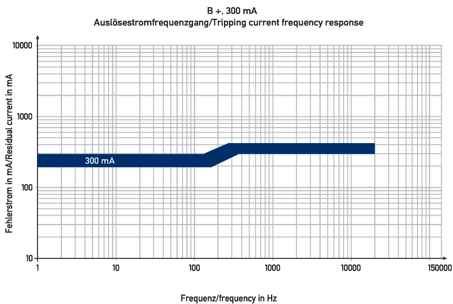
Curva característica B+ 300 mA
