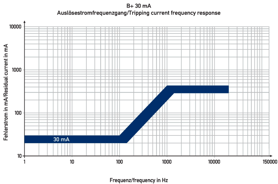
Curva característica B+ 30 mA
