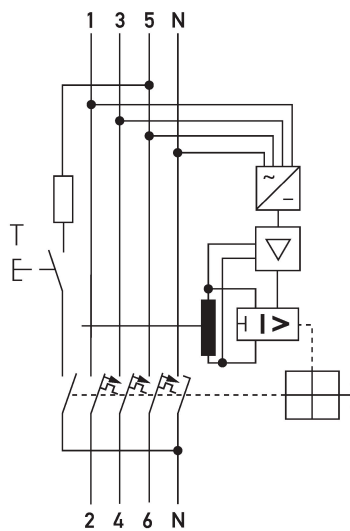
Anschlussschema DRCBO 4 Typ B NK, 3+N-polig
