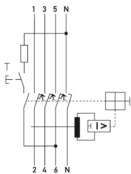
Ejemplo de cableado Combinaciones de interruptores diferenciales e interruptores magnetotérmicos DRCBO 4 C25/0,03/3N-A
