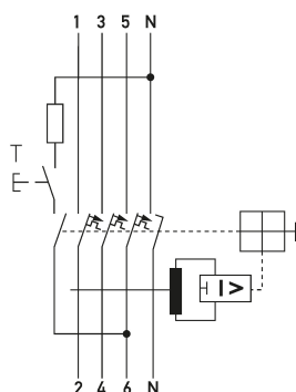
Schaltungsbeispiel FI-/LS-Kombinationen DRCBO 4 B25/0,03/3N-A
