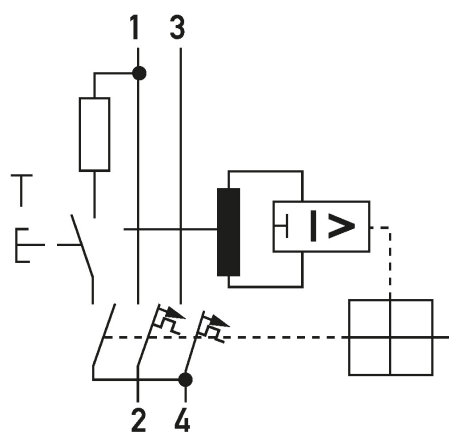
Esquema de conexiones DRCBO 2 tipo A KV, 2 polos
