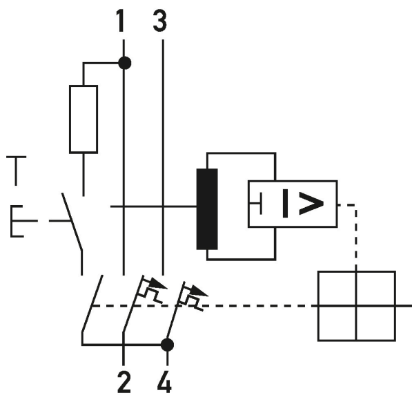
Esquema de conexiones DRCBO 2 tipo A, 2 polos
