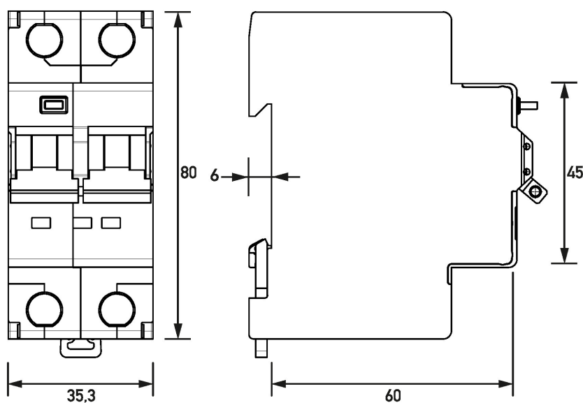
Dibujo acotado (Vista de grupos)
