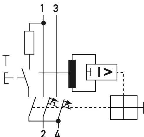
Esquema de conexiones
