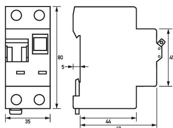
Dibujo acotado Combinaciones de interruptores diferenciales e interruptores magnetotérmicos DRCBO 3 C16/0,01/1N-AC
