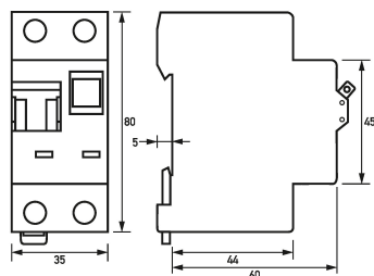
Dibujo acotado Combinaciones de interruptores diferenciales e interruptores magnetotérmicos DRCBO 3 Co6/0,03/1N-AC
