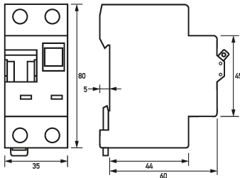
Dibujo acotado Combinaciones de interruptores diferenciales e interruptores magnetotérmicos DRCBO 3 D20/0,03/1N-F
