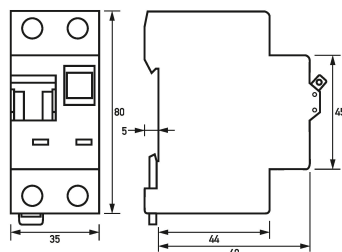
Maßzeichnung FI-/LS-Kombinationen DRCBO 3 C20/0,10/1N-F
