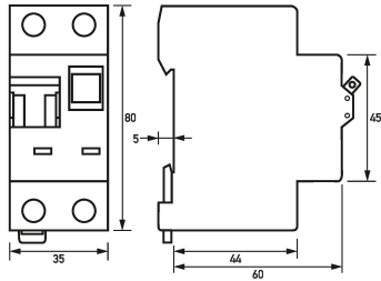
Dibujo acotado Combinaciones de interruptores diferenciales e interruptores magnetotérmicos DRCBO 3 C25/0,03/1N-F
