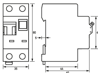
Dibujo acotado Combinaciones de interruptores diferenciales e interruptores magnetotérmicos DRCBO 3 C10/0,03/1N-A V110
