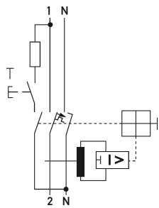
Ejemplo de cableado Combinaciones de interruptores diferenciales e interruptores magnetotérmicos DRCBO 3 tipo A, 1 polo + N
