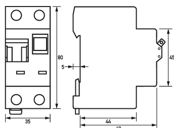
Dibujos acotados de combinaciones de interruptores diferenciales e interruptores magnetotérmicos DRCBO 3 tipo A, 1 polo + N
