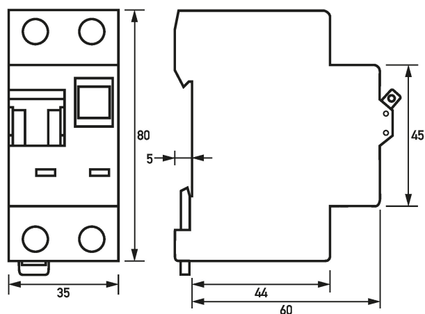
Dibujo acotado (Vista de grupos)
