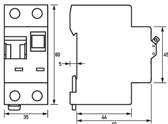
Maßzeichnung FI/LS-Kombinationen DRCBO 3 B20/0,10/1N-A
