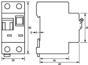
Dibujo acotado Combinaciones de interruptores diferenciales e interruptores magnetotérmicos DRCBO 3 Bo6/0,01/1N-A
