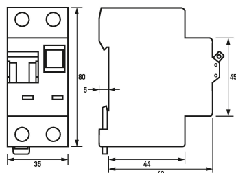
Dibujo acotado Combinaciones de interruptores diferenciales e interruptores magnetotérmicos DRCBO 3 C13/0,30/1N-A
