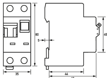
Maßzeichnung FI-/LS-Kombinationen DRCBO 3 Typ A, 1+N-polig
