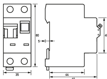
Dibujo acotado Combinaciones de interruptores diferenciales e interruptores magnetotérmicos DRCBO 3 C16/0,03/1N-A
