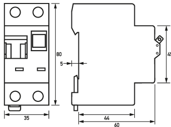
Dibujo acotado Combinaciones de interruptores diferenciales e interruptores magnetotérmicos DRCBO 3 B16/0,30/1N-A
