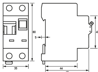
Maßzeichnung FI-/LS-Kombinationen DRCBO 3 B20/0,03/1N-A
