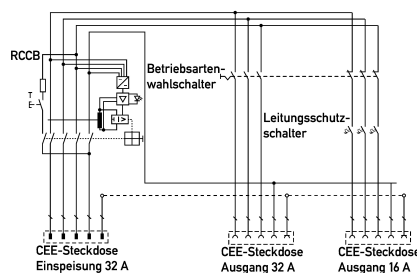
Esquema de conexiones
