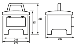
Dibujo acotado Vista de grupos
