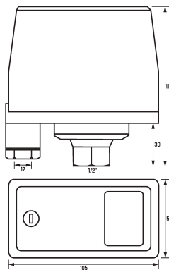
Dibujo acotado Vista de grupos
