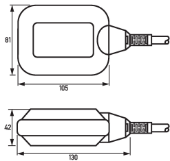
Dibujo acotado Interruptores de flotador Champ 1 GS-F 05 m
