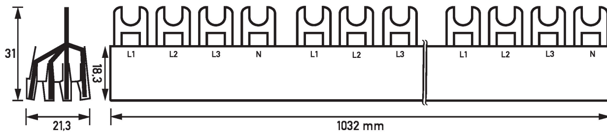
Dibujo acotado Barras para interruptores diferenciales/interruptores magnetotérmicos recortables a medida (Vista de grupos)
