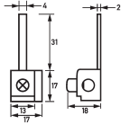
Maßzeichnung Gruppenansicht
