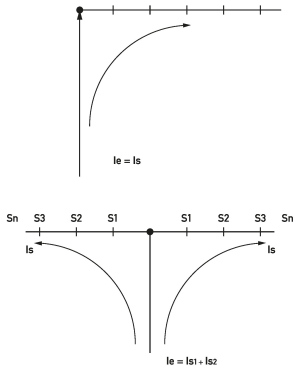
Diagramas Materiales de cableado BG4.5.16
