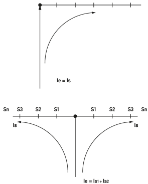
Diagramas Materiales de cableado EV-S G 1.12.70
