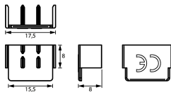
Dibujo acotado Vista de grupos
