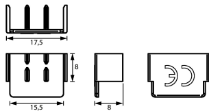
Maßzeichnung Endkappen EK-3/10/16
