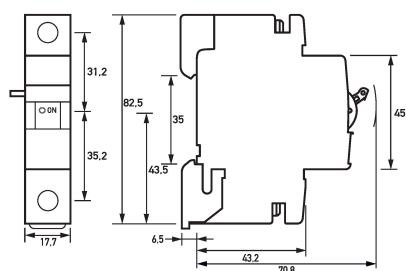
Maßzeichnung Arbeitsstromauslöser DASA 12
