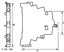
Dibujo acotado Vista de grupos
