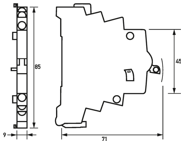
Maßzeichnung DHi für DLS 6 (Gruppenansicht)
