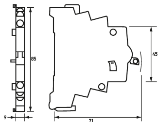
Dibujo acotado Interruptores auxiliares DHi 5
