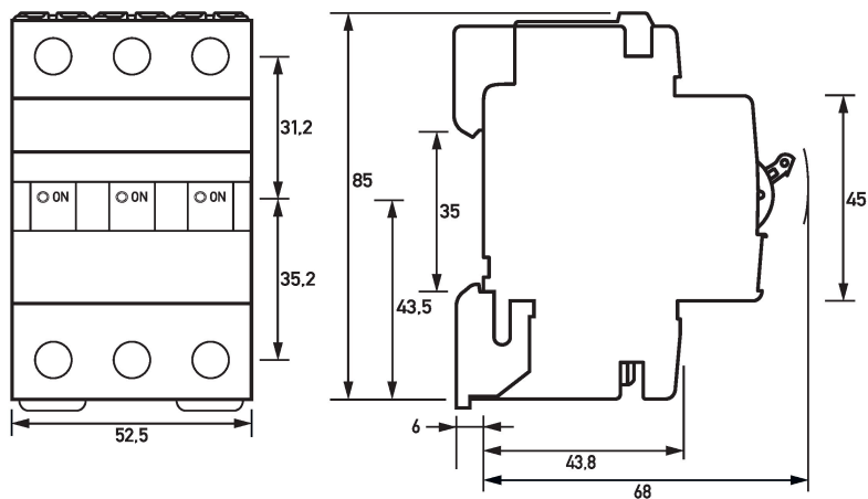
Maßzeichnung DLS 6hsl, C-Charakteristik, dreipolig (Gruppenansicht)
