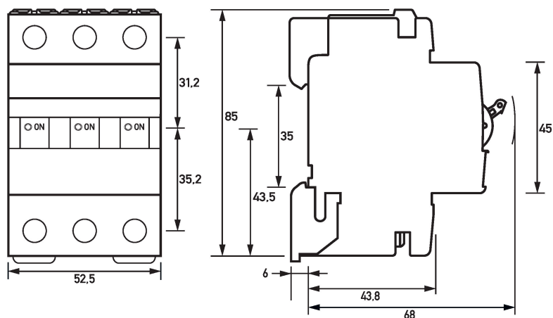
Dibujo acotado DLS 6hsl, característica C, tres polos (Vista de grupos)
