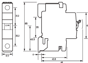
Maßzeichnung Gruppenansicht
