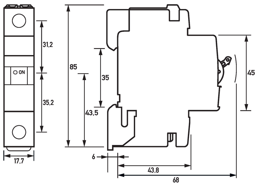
Maßzeichnung DLS 6hsl, C-Charakteristik, einpolig (Gruppenansicht)
