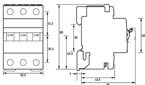
Maßzeichnung Gruppenansicht
