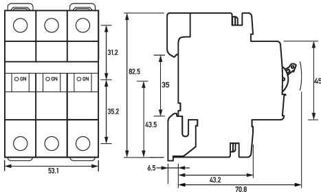
Dibujo acotado Interruptores magnetotérmicos DLS 6i Z13-3
