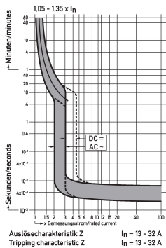
Diagramas Interruptores magnetotérmicos DLS 6i Z13-3
