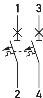
Anschlusschema DLS 6i, Z-Charakteristik, zweipolig, 10kA
